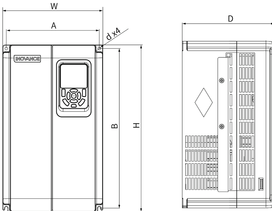
Модели размера T5-T6
