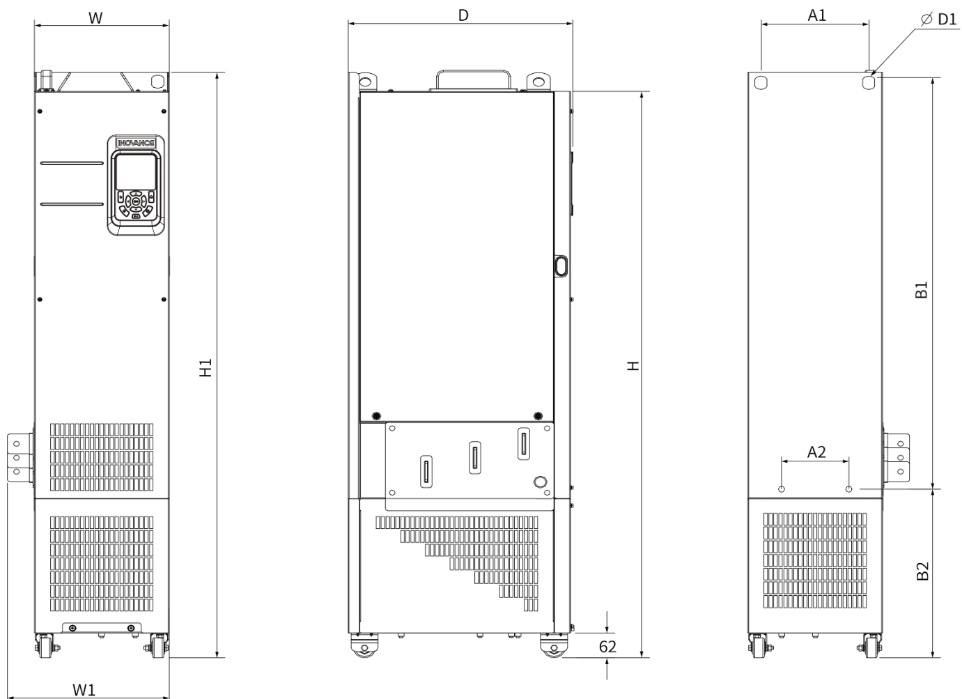
Модели размера Т10-Т12 со встроенным выходным дросселем
