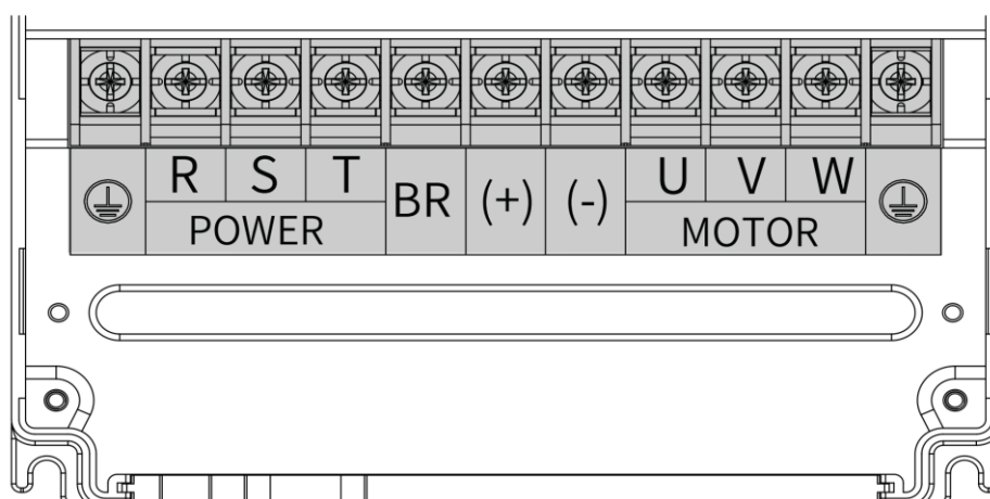
Расположение клемм трёхфазных моделей размера T5-T8
