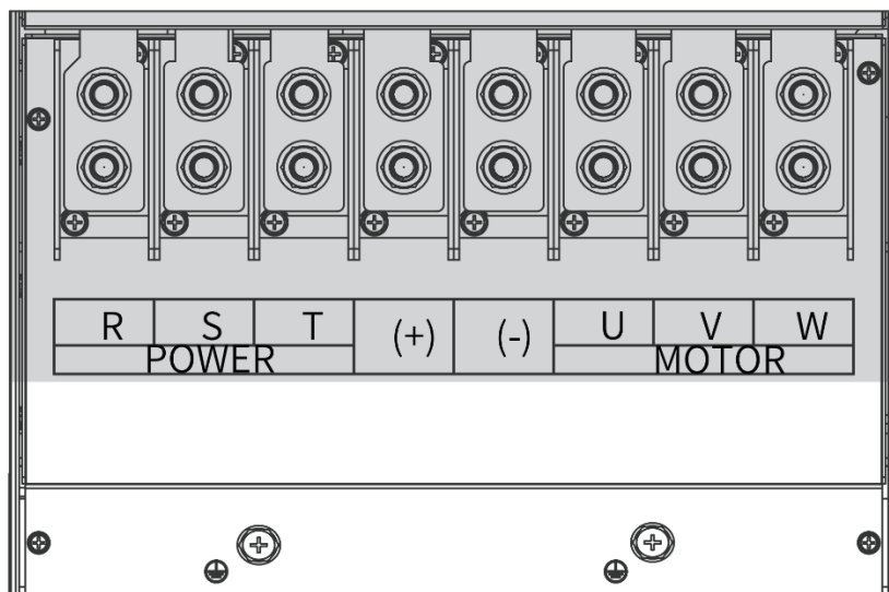
Расположение клемм трёхфазных моделей размера T9
