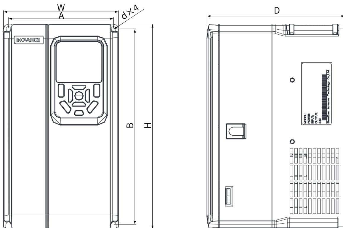
Модели размера T1-T4
