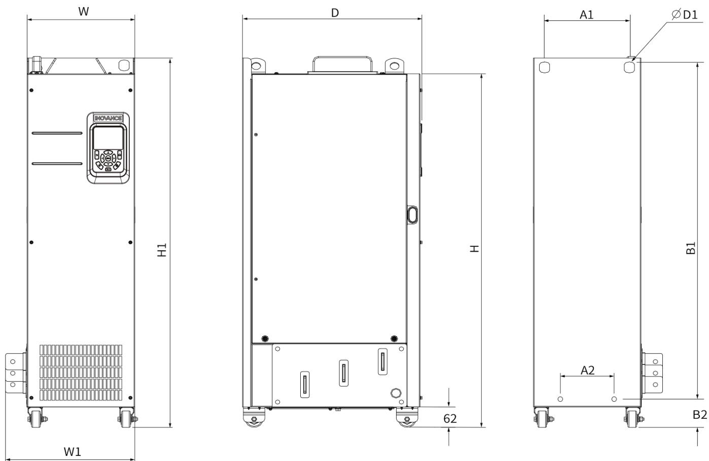
Модели размера T10-T12 без встроенного выходного дросселя
