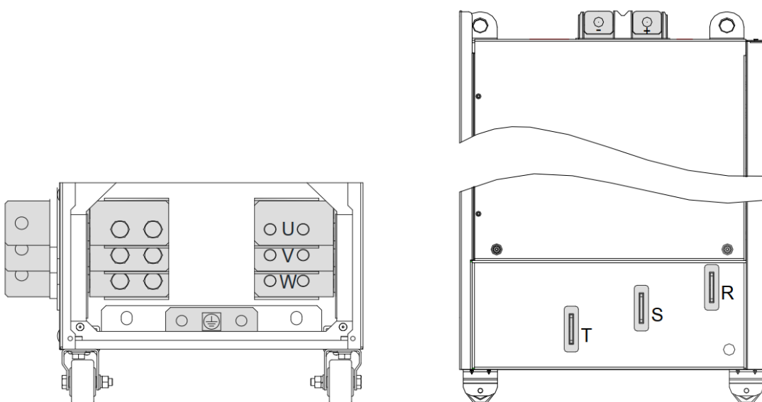
Вид спереди
