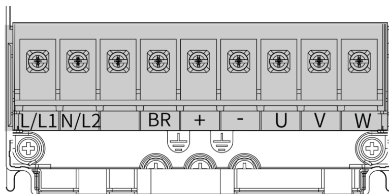
Расположение клемм однофазных моделей размера T2
