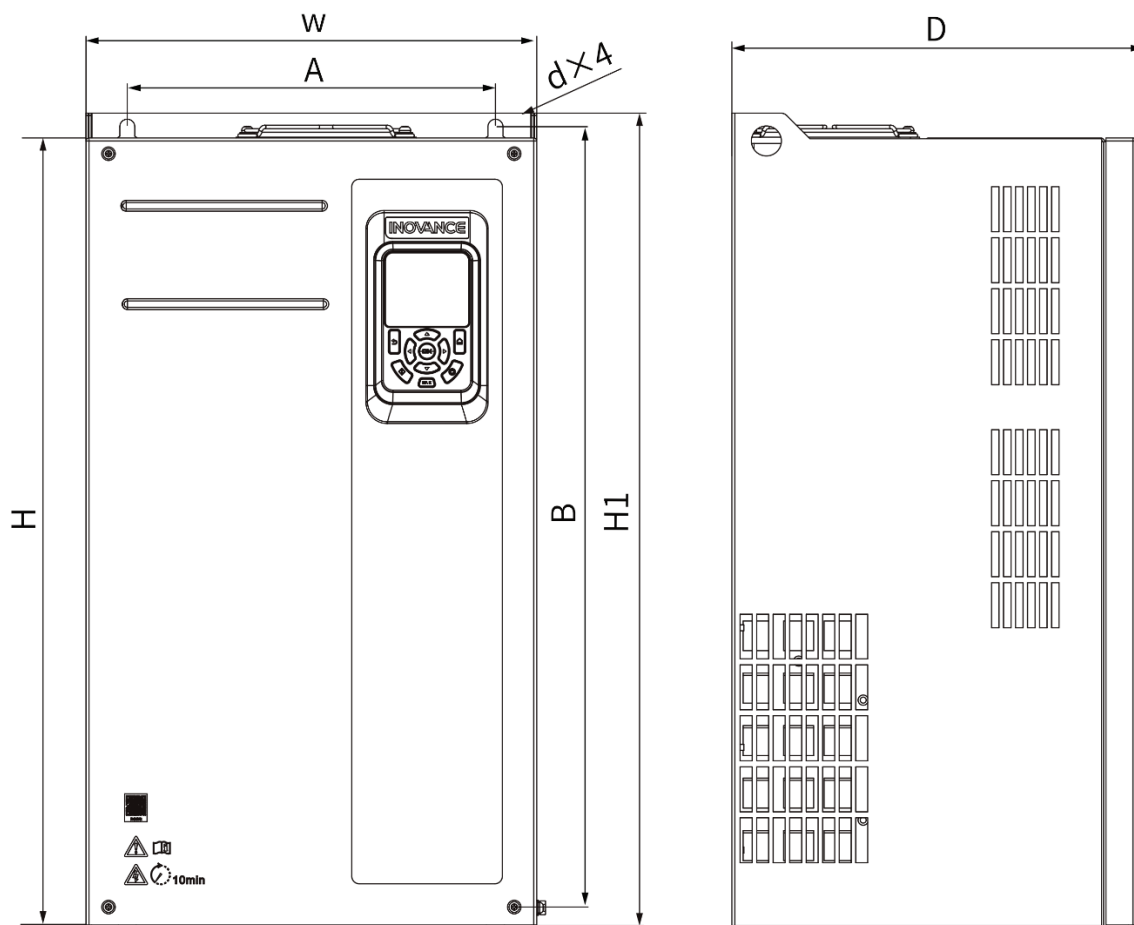
Модели размера Т7-Т9
