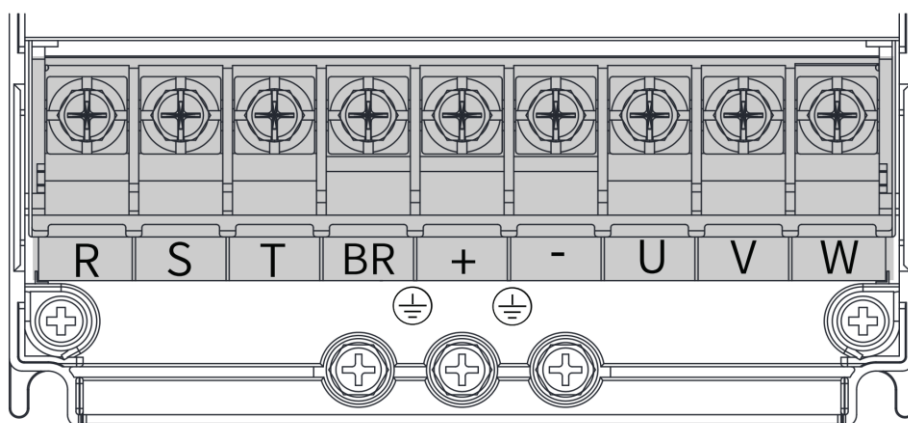
Расположение клемм трёхфазных моделей размера T1-T4
